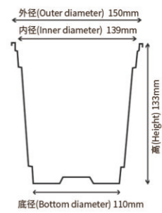
⑥ 双色花盆(Double Color Pot) 150x133mm
