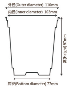
⑩ 双色花盆(Double Color Pot) 110x97mm
