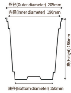
① 双色花盆(Double Color Pot) 205x186mm
