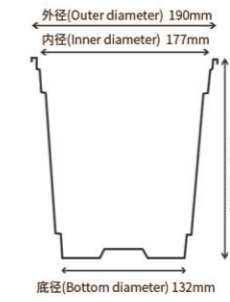
② 双色花盆(Double Color Pot) 190x170mm
