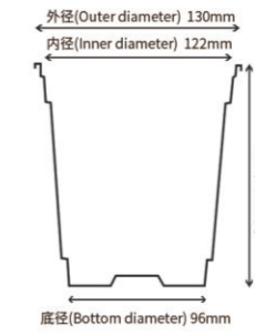
⑧ 双色花盆(Double Color Pot) 130x114mm
