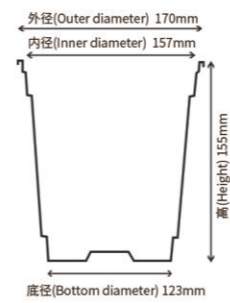
④ 双色花盆(Double Color Pot) 170x155mm
